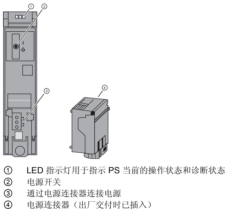
图 2-2 PS 25W 24VDC（无前盖板）和电源连接器视图
