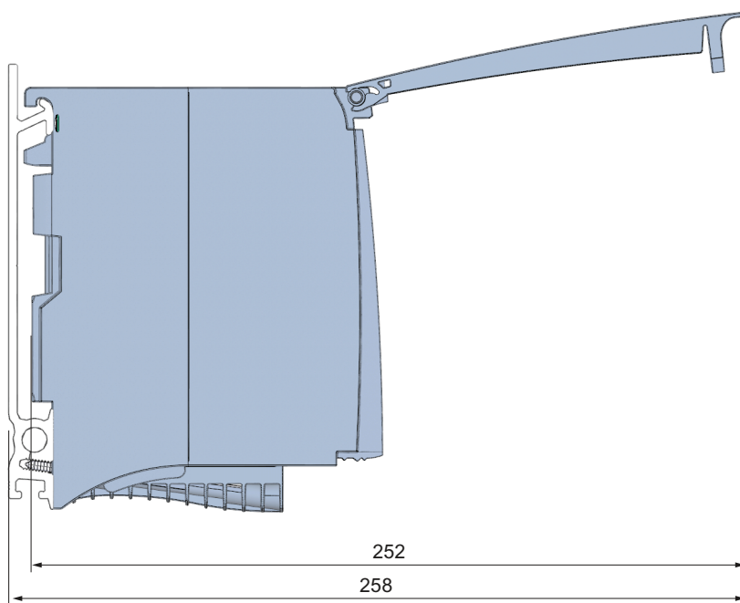
图 A-2 PS 25W 24VDC 模块打开前盖板时侧视图的尺寸图
