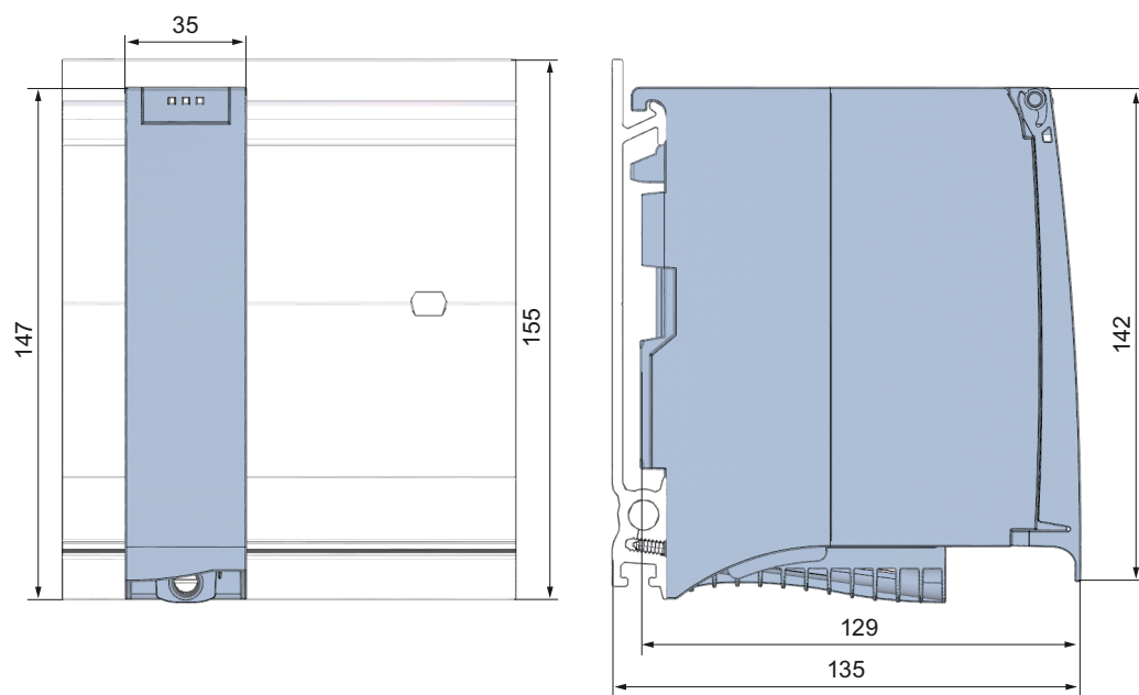
图 A-1 PS 25W 24VDC 模块的尺寸图
