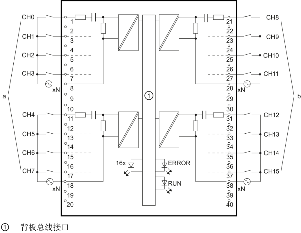
图 3-1 方框图和端子分配
