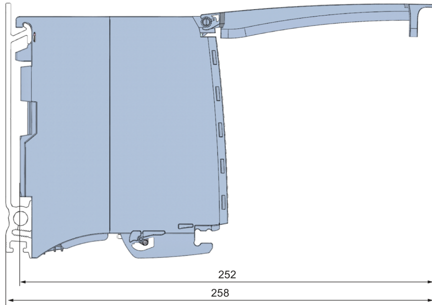
图 A-2 DI 16x24VAC BA 模块的尺寸图，带开放式前盖的侧视图
