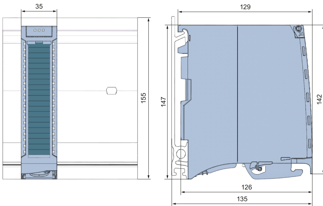
图 A-1 DI 16x24VAC BA 模块的尺寸图
