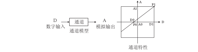
图 3-4 IVC1-5AM 的输出通道特性示意图
