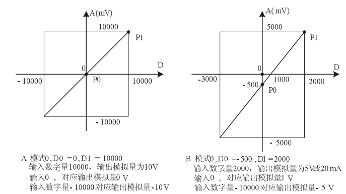
图 3-6 输出通道特性更改举例
