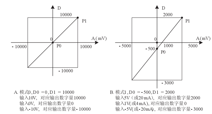
图 3-3 输入通道特性更改举例
