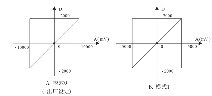
图 3-2 输入通道各种模式默认的通道特性
