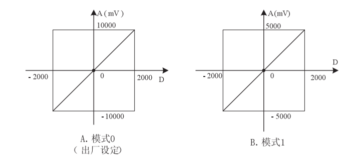
图 3-5 输出通道各种模式默认的通道特性
