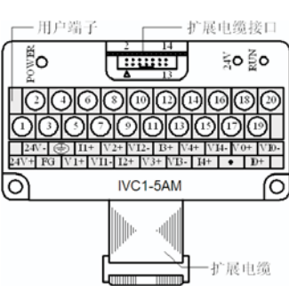
图 1-2 模块接口端子图
