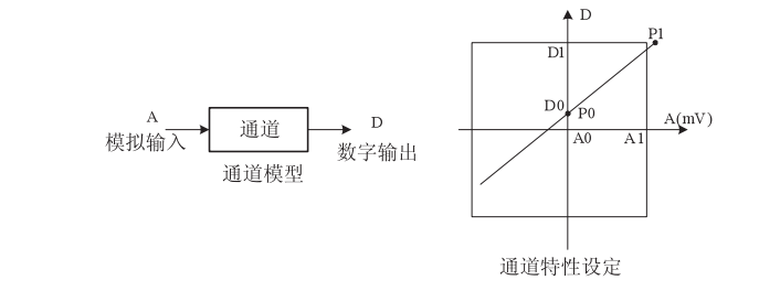
图 3-1 IVC1-5AM 的输入通道特性示意图
